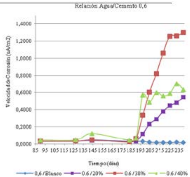
Figura 4. Variación de la velocidad de corrosión con respecto al tiempo, para probetas con relación a/c igual a 0,6
