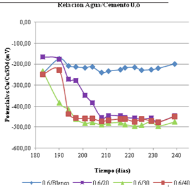
Figura 2. Variación del potencial durante el tiempo de exposición de las probetas de relación a/c 0,6.
