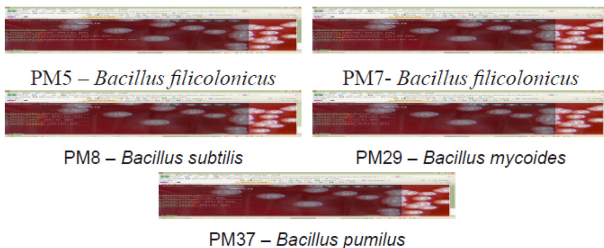
Figura 2. Especies bacterianas pertenecientes al género Bacillus
