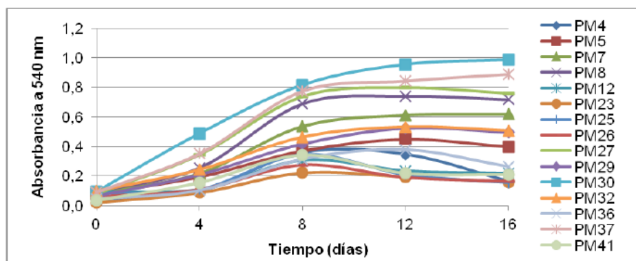
Figura 1. Crecimiento bacteriano en diesel determinado por espectrofotometría a \lambda = 540 nm.
