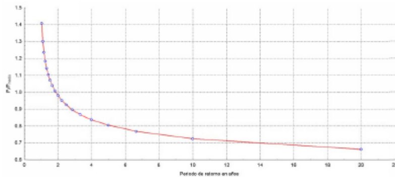
Figura 6.- Curva de crecimiento regional de la región homogénea N° 6. P_{media} = 1154.81 \text{ mm/año}
